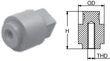
80-100 HP
