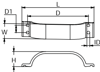
150 / 200 HP
