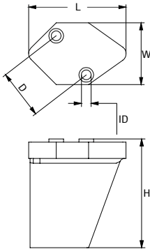
YAMAHA 9,9 - 15 HP
