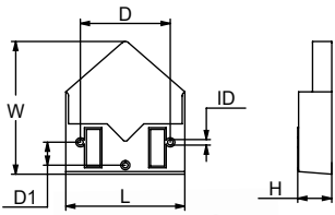
V8
